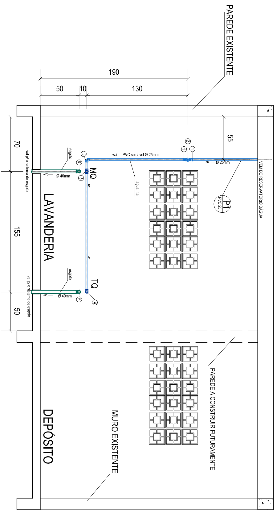
CASA PASSAGEM - VISTA A Escala 1:30
